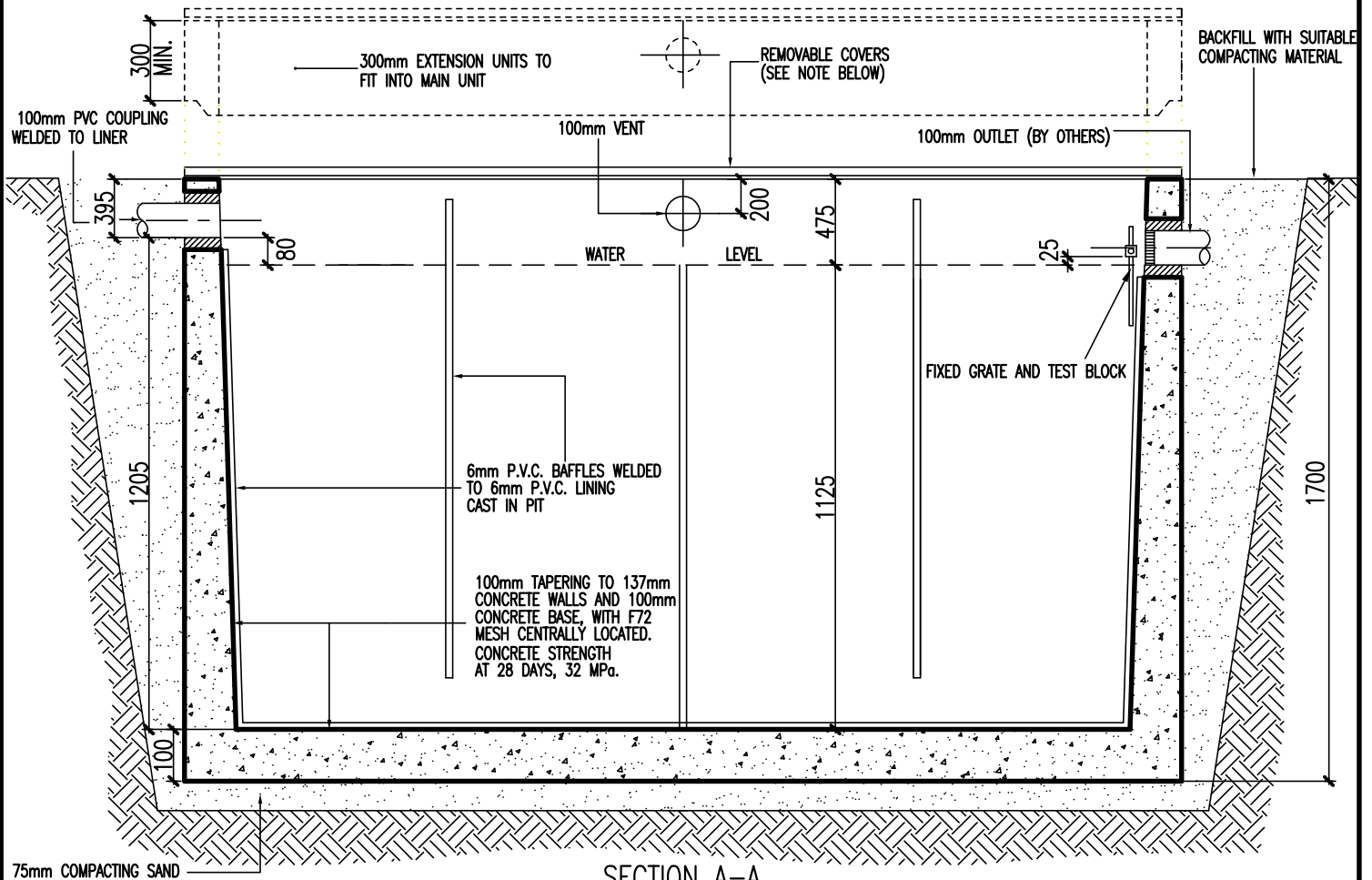
SECTION A-A 2575
