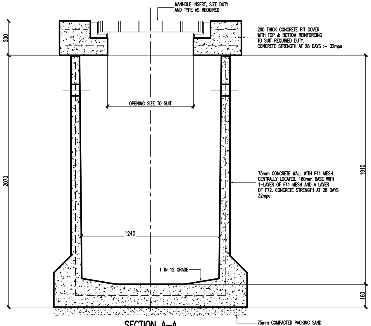
SECTION A-A
