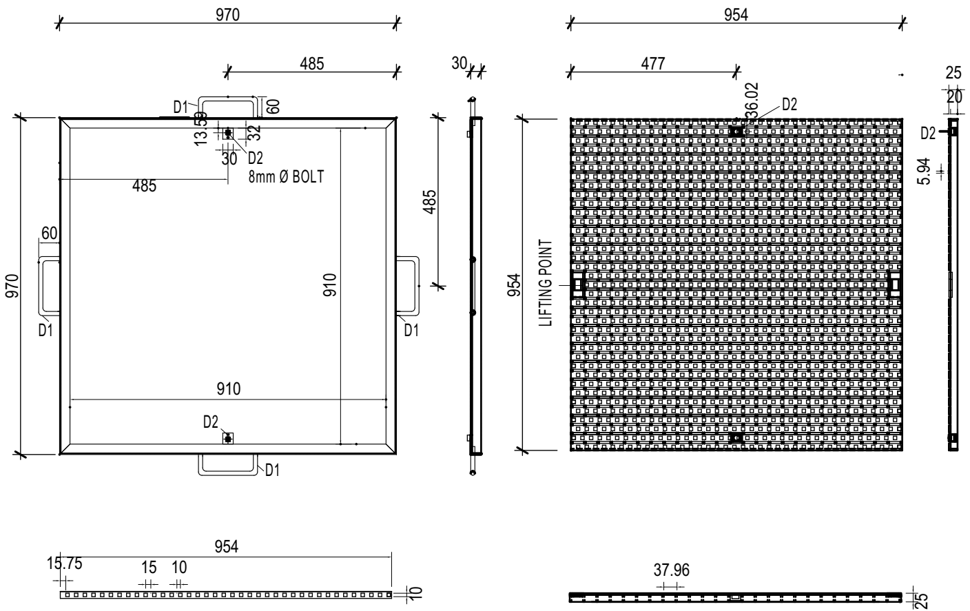
NON SLIP FLAT BAR DETAIL
