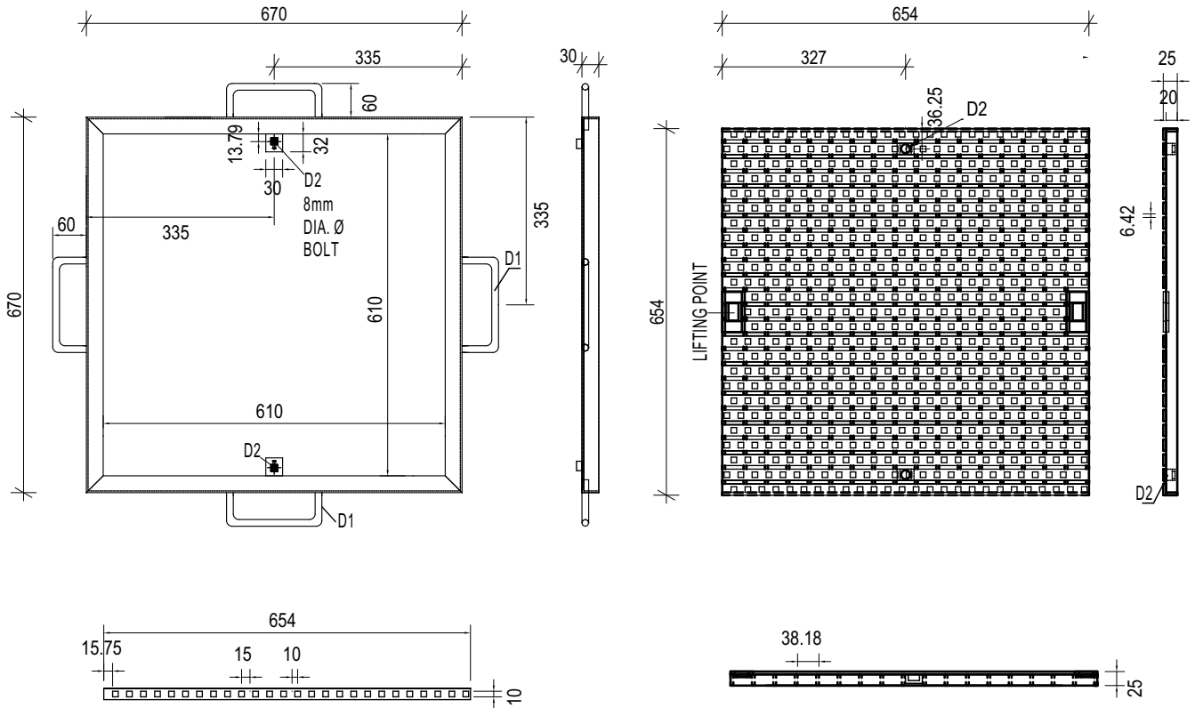
NON SLIP FLAT BAR DETAIL
