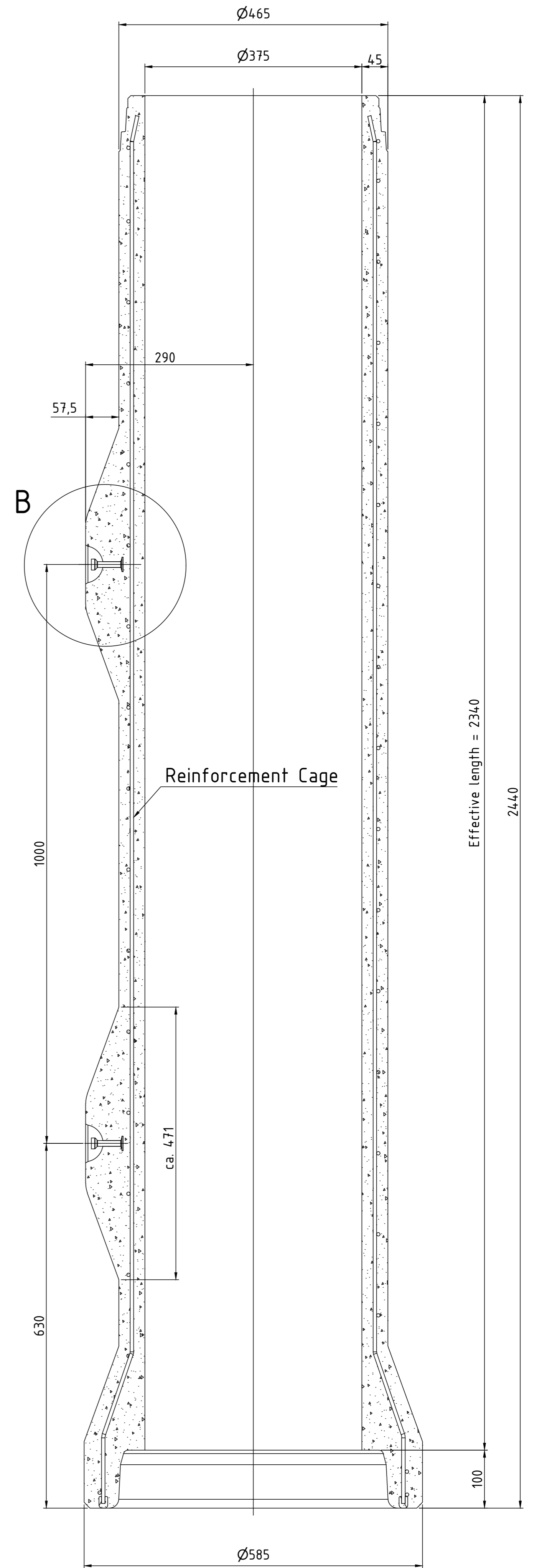
Section A-A
