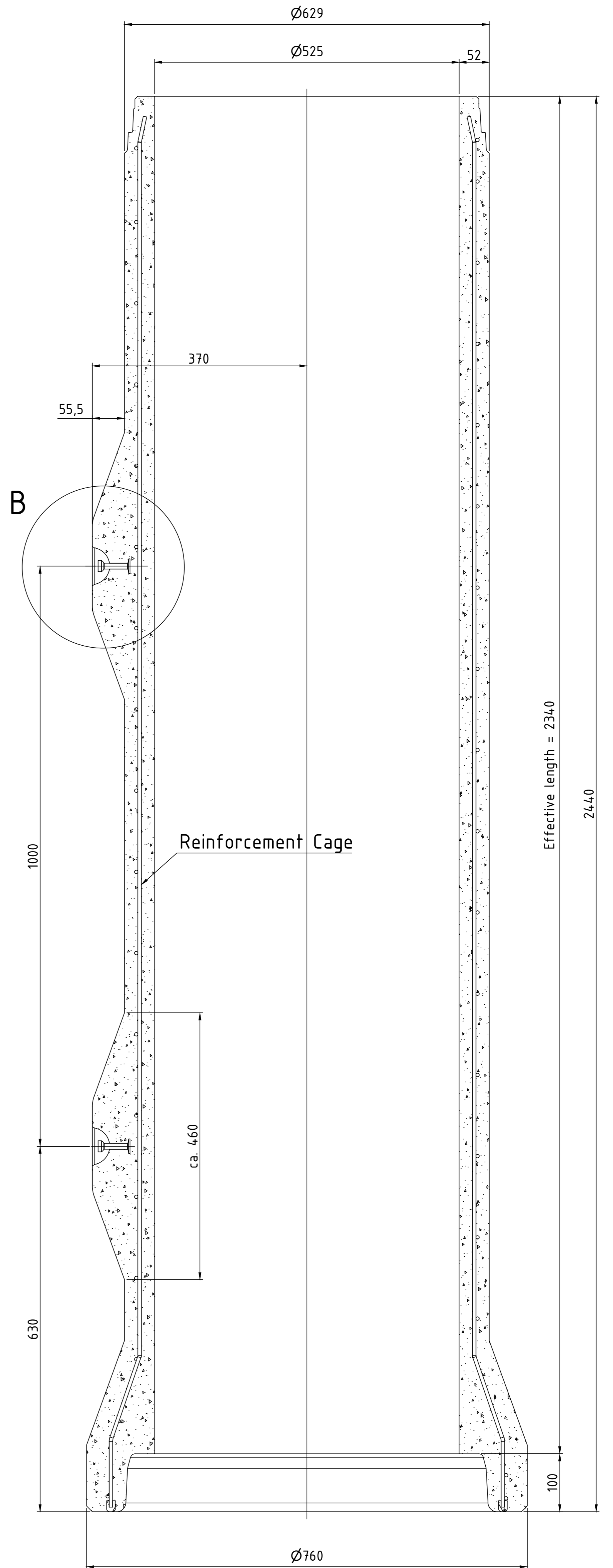
Section A-A
