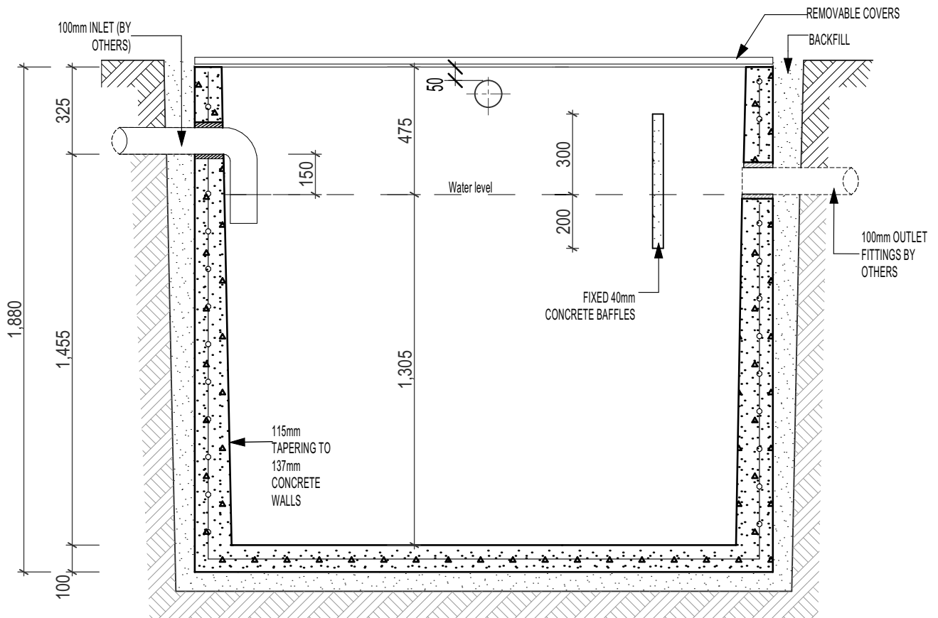
SECTION A-A
