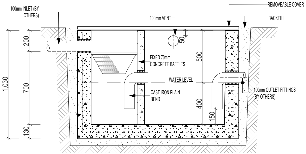
SECTION A-A
