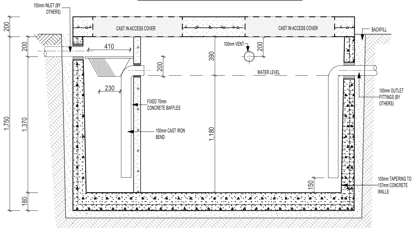
SECTION A-A
