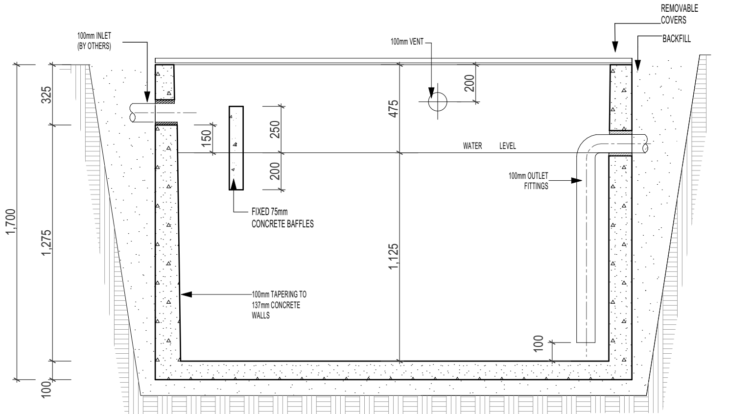
SECTION A-A
