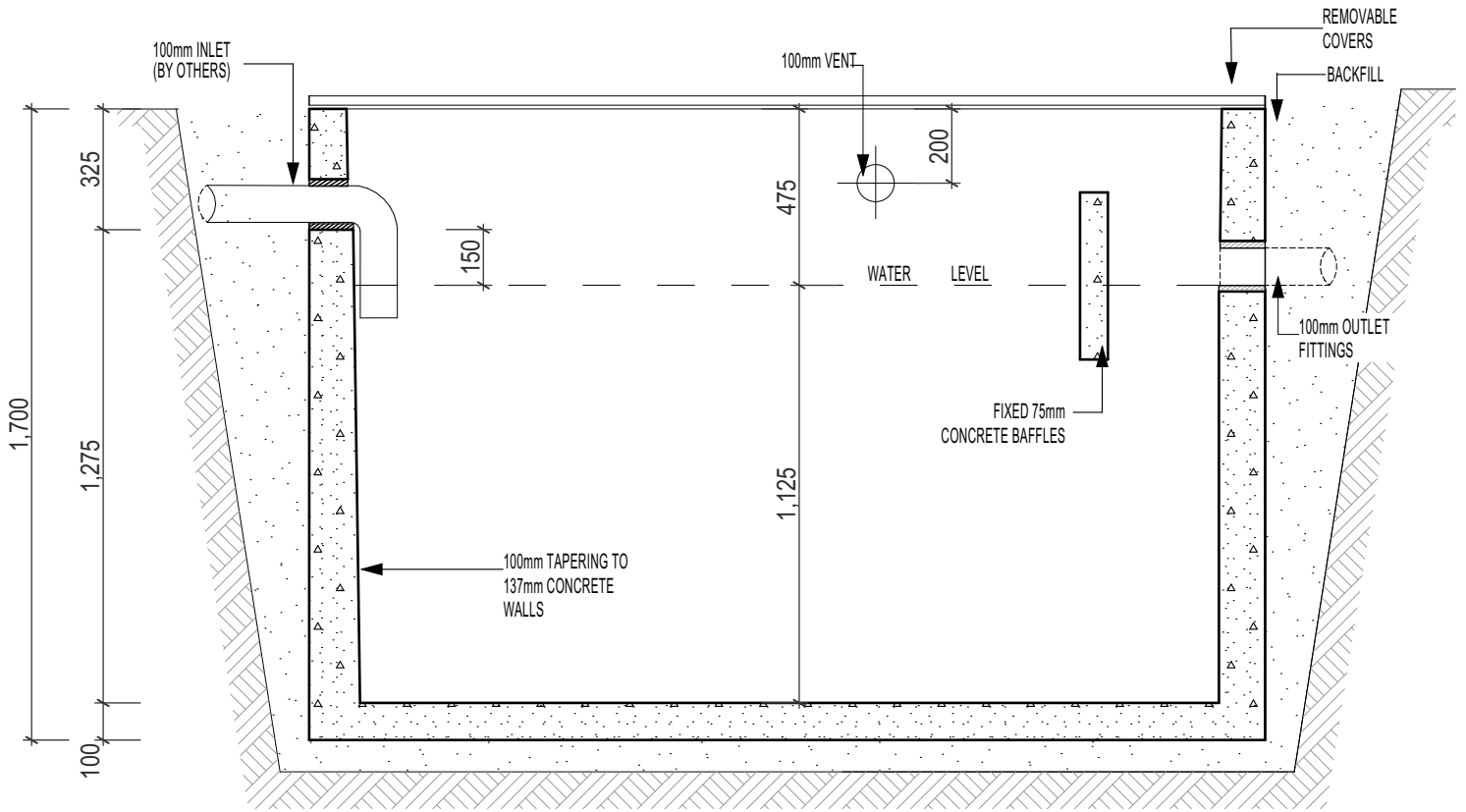
SECTION A-A
