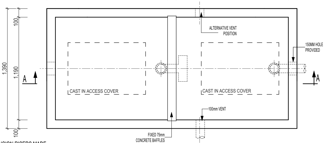
PLAN WEIGHT 7000KG
